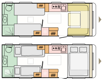
613 UT L 6761 (mm) | W 2460 (mm) | 4
