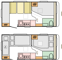
472 PK L 5174 (mm) | W 2300 (mm) | 6
