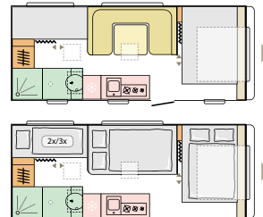
573 PT L 6365 (mm) | 6 W 2460 (mm)
