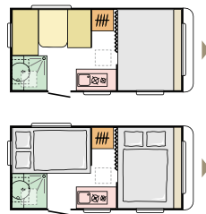
400 PS L 4492 (mm) | W 2090 (mm) | 4
