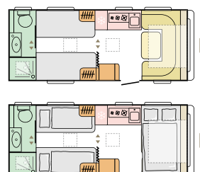
572 UT L 6400 (mm) | 4 W 2299 (mm)
