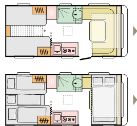
502 UL L 5725 (mm) | 5 W 2299 (mm)
