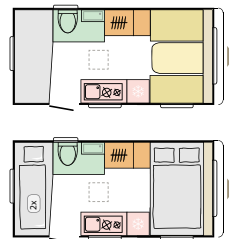
400 DK L 4492 (mm) | W 2090 (mm) | 4
