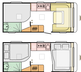
522 UP L 5910 (mm) | 4 W 2299 (mm)
