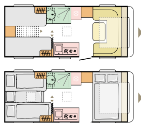
542 UL L 6150 (mm) | 5 W 2299 (mm)
